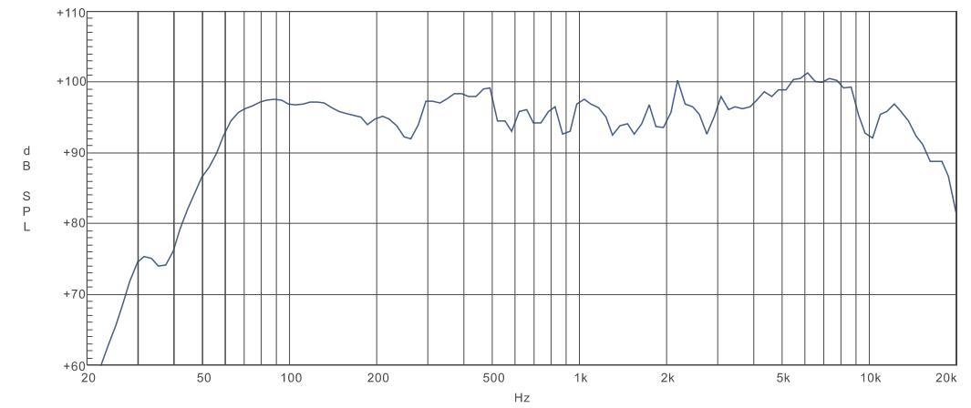
TPS i12H
