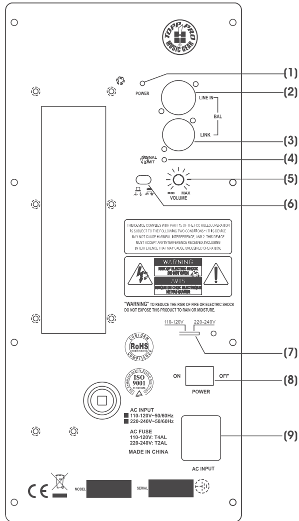
TPS i10HA/i12HA/i15HA/i28HA/i210HA
